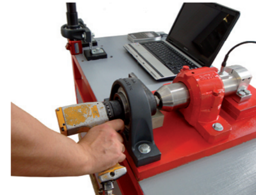
Hochmomentschrauber-Test
